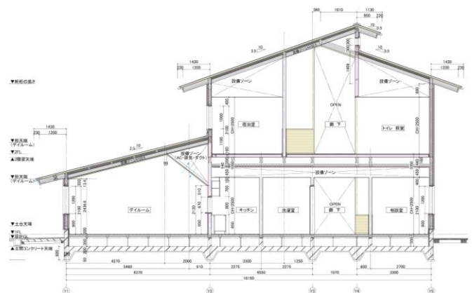
④事務局モデル案 矩計図
