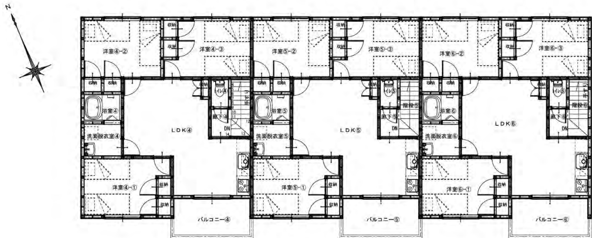
2 階平面図
