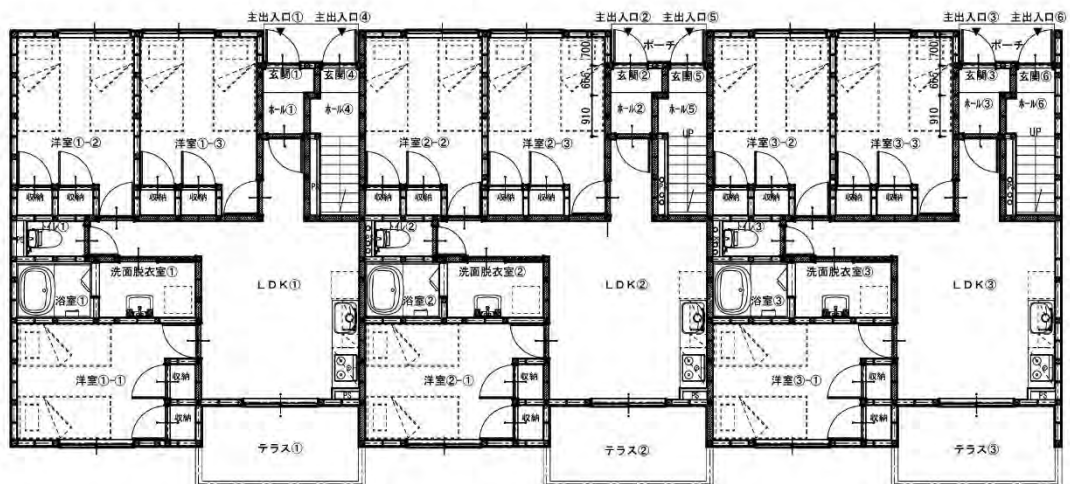
1 階平面図
