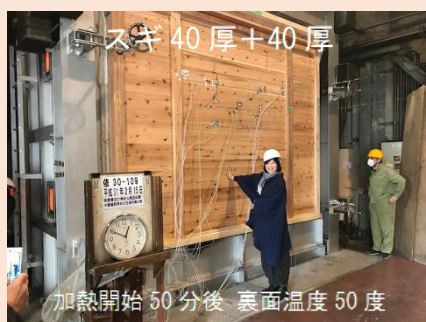
落とし込み板壁の加熱実験の様子 (一社)日本板倉建築協会)
